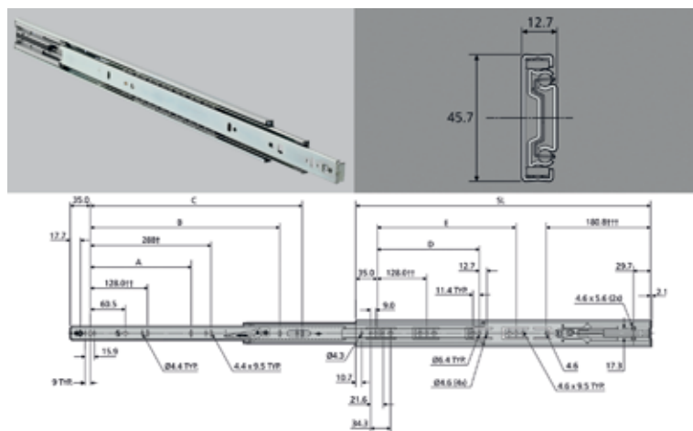
Glissière Accuride type 3832B
