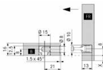
Raidisseur pour tiroirs pour Scala
