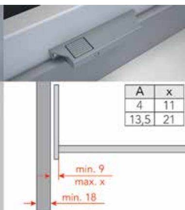
Entraîneur pour face - PVC gris
